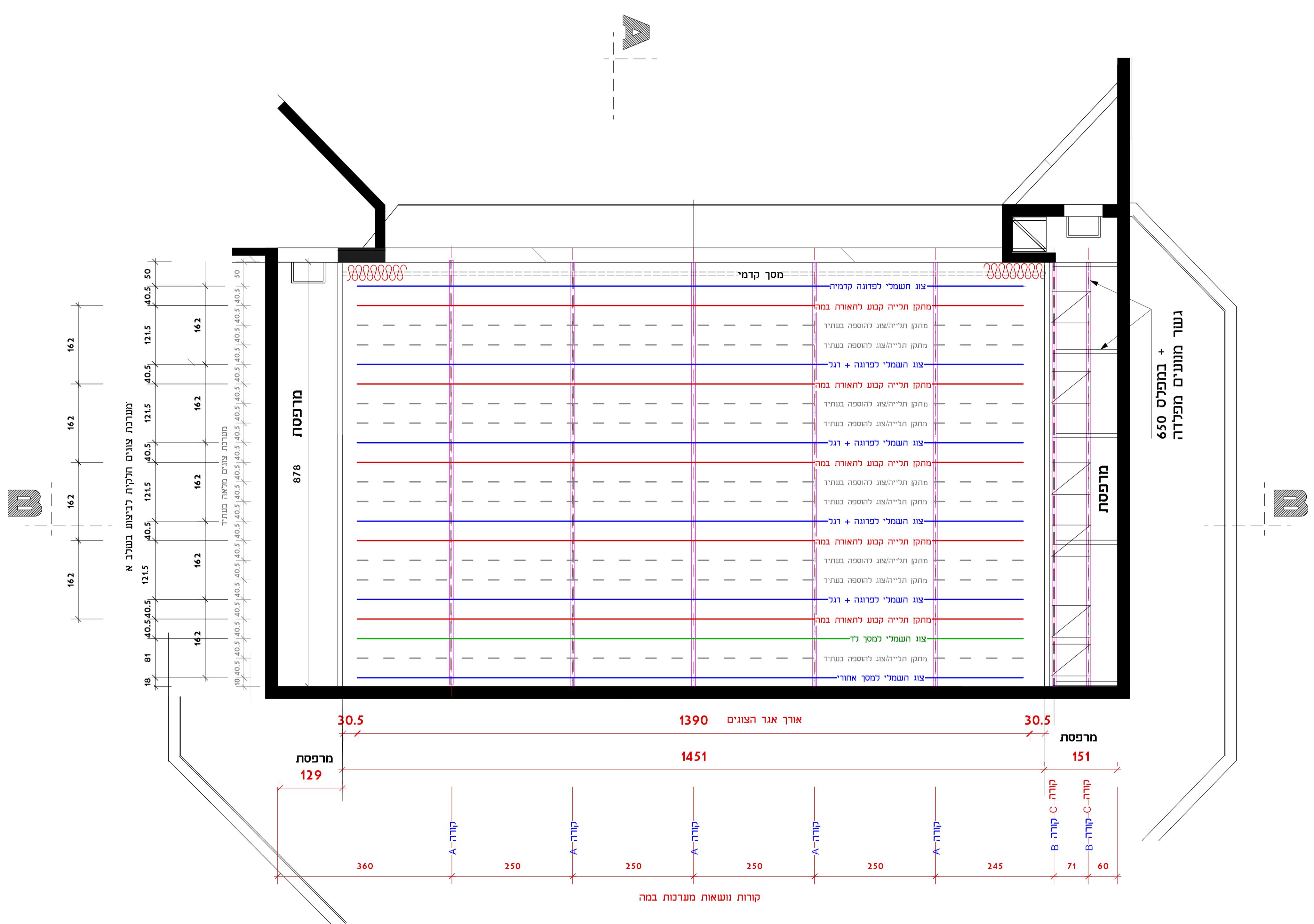
+ תוכנית מערכת הצוגים בבמה 1:50
