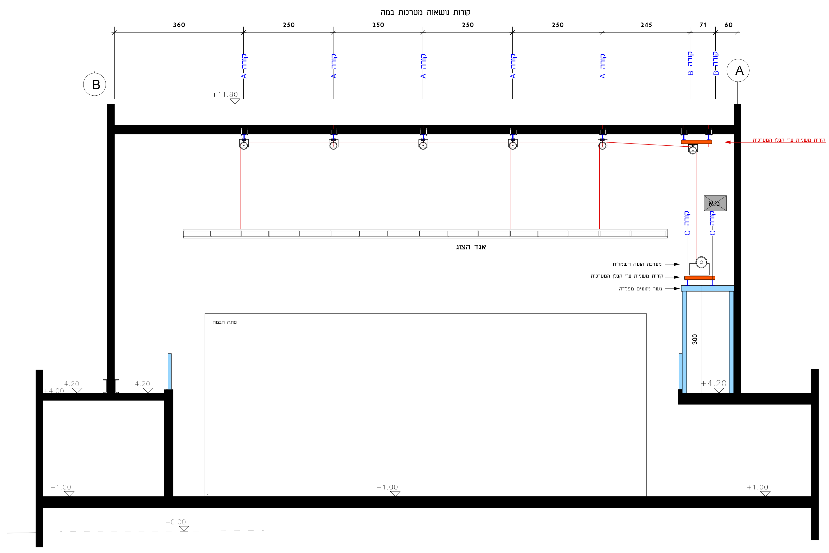
חתך B-B - צוגים השמליים 1:50
